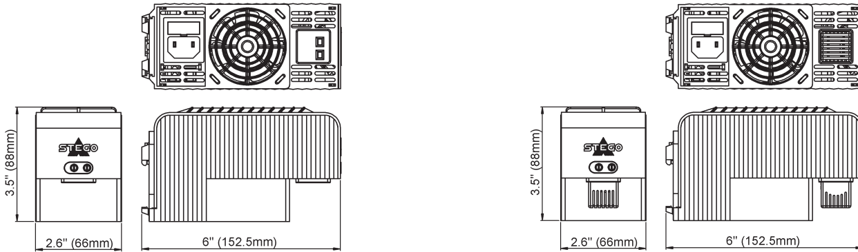
CS 032 Fan Heater
